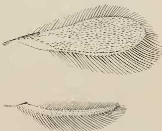
Fig. 20.— A. ovijentatus , wing.
